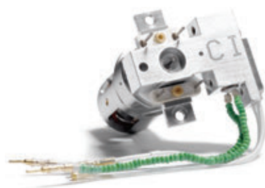
5977/5975/5973/7000 Ion Source
